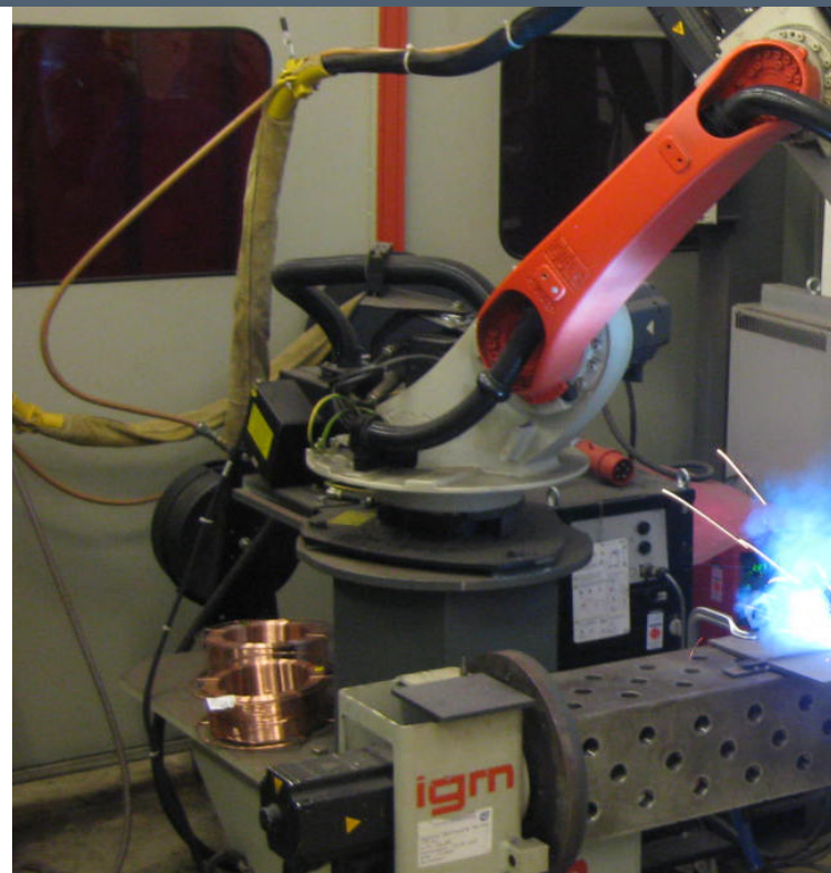
Robotertraining mit Prüfung nach DIN EN ISO 14732
