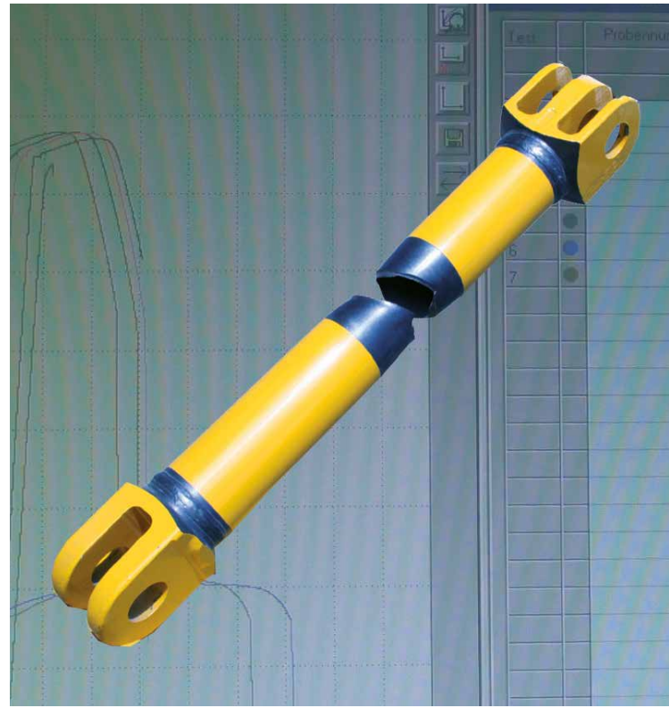
Zugprobe einer Gabel-Holmrohr-Verbindung
