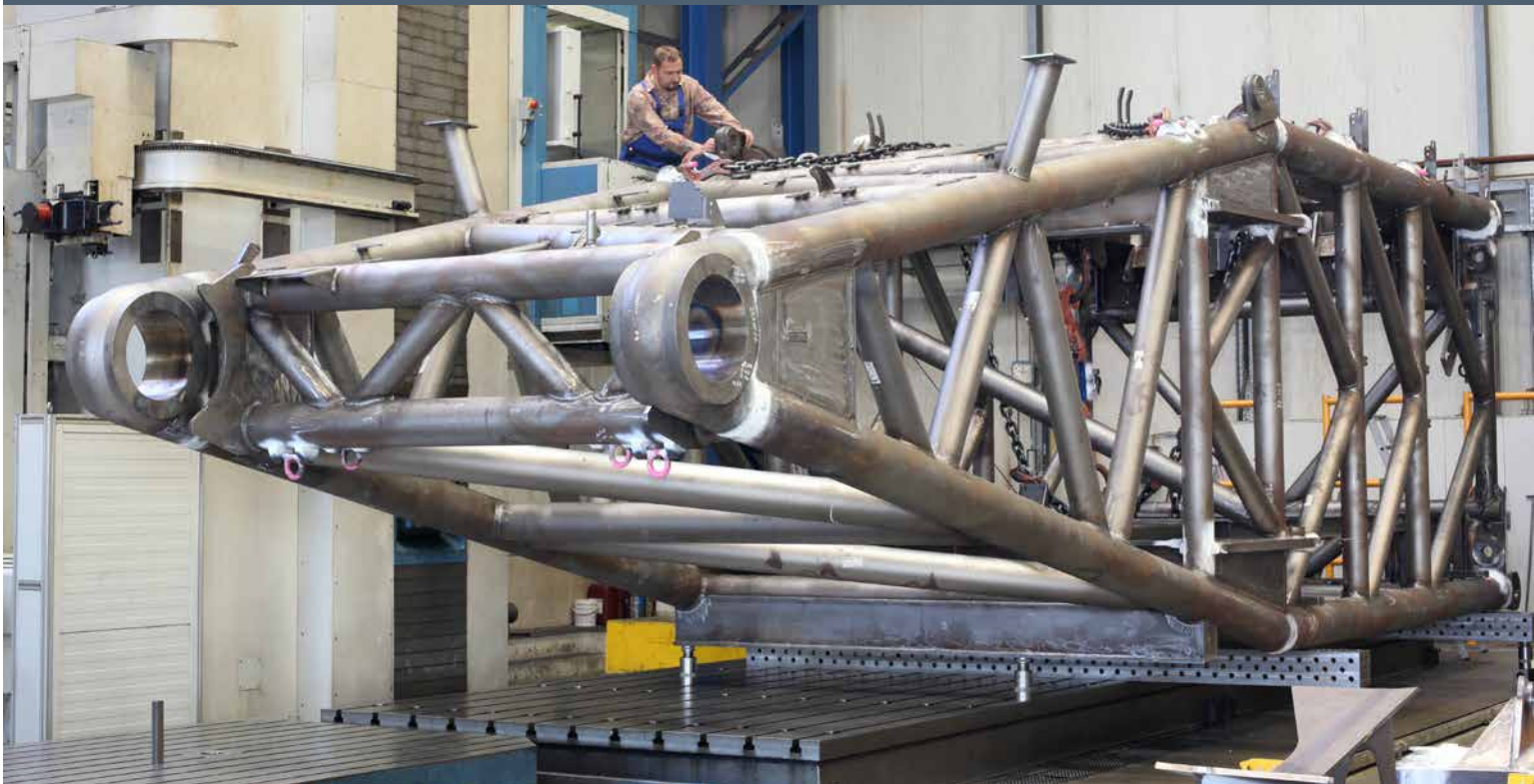
Gitterteil für Raupenkran
